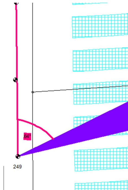
Abbildung 4.2: Blickwinkelanalyse DEG 31 (lila: Reflexionsstrahlen, pink: Fahrtrichtung)
