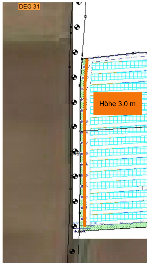
Abbildung 5.1: Lage Blendschutzzaun
